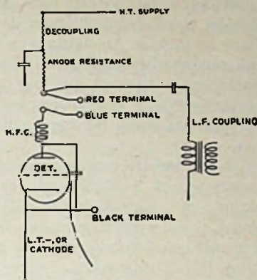
Fig. 1. Schakeling der detectorlamp met „stroomlozen” transformator. De roode kleur (red terminal) en de blauwe kleur (blue terminal) van het filter worden op de aangegeven plaatsen verbonden. De zwarte kleur (black terminal) komt aan kathode. De pijl geeft een capaciteit van 300 \mu\mu F tusschen plaat en kathode aan, welke gewenscht is als men de hfr. smoorspoel blijft gebruiken.
