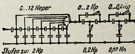
Fig. 1. Principeschema van een H.F.-ijklijn.
