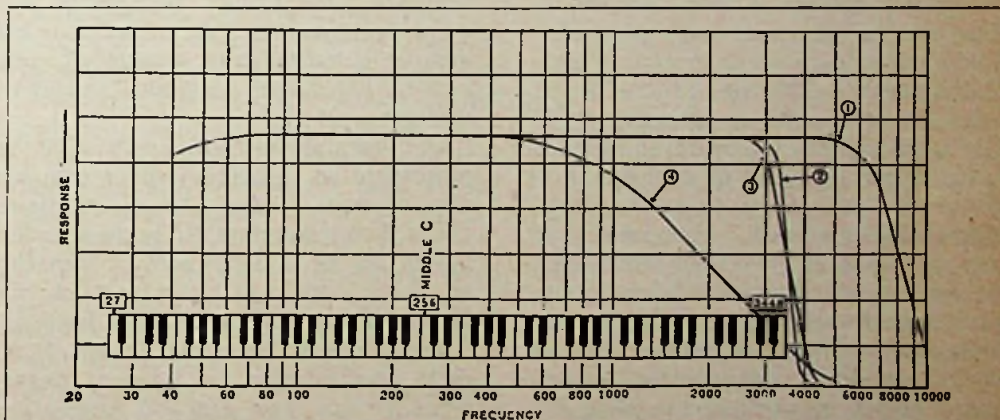
Fig. 2. Eenige krommen, welke de werking van het filter aangeven. Kromme 1 is de weergavekromme van een goeden e.d. luidspreker, die tot 8000 en 9000 hertz gaat. Tracht men met een condensator over transformator of luidspreker hinderlijke giltonen te laten verdwijnen, dan ontstaat een weergave volgens kromme 4, die alle voordeelen van den goeden luidspreker te niet doet; de afsnijding begint al bij 500 hertz, wanneer men 4000 Hz onhoorbaar wil maken. Met het vroeger besproken dubbele Kinox-filter ontstaat kromme 2, die een zeer scherpe afsnijding voorstelt, met zoo gering mogelijk verlies van hoge tonen. Het nieuwe enkelvoudige filter levert met geheel ingeschoven kern kromme 3 op; deze is iets minder scherp, maar toch nog heel goed en de afsnijding kan bovendien meer naar rechts verschoven worden.
